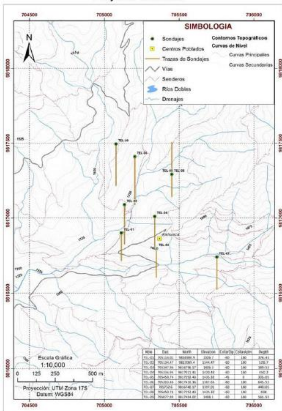
Mapa VI. Mapa de ubicación de los sondajes exploratorios del Proyecto Telimbela – Sector Ashcoaca.
