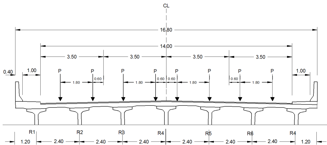
Figura 7.18: Sección transversal y ubicación de vehículos para momentos tramo 1. Fuente: Autores.
