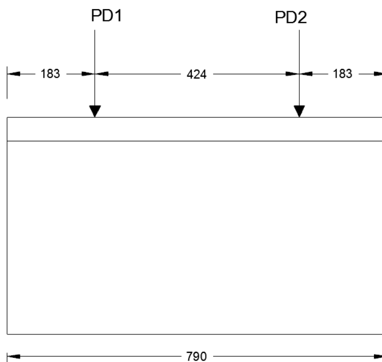
Figura 4.17: Ubicación de cargas muertas Pila 2. Fuente: Autores.
