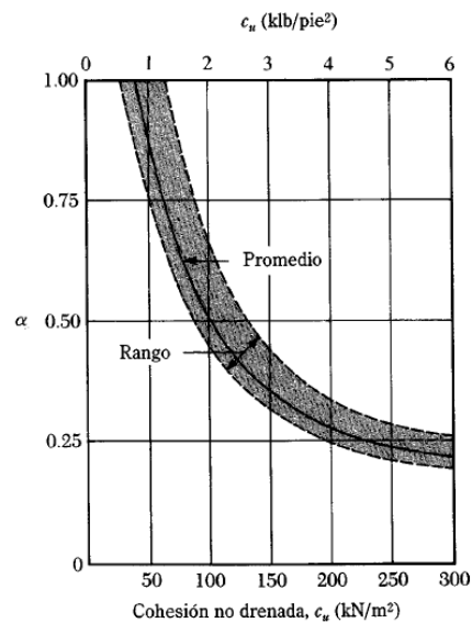
Figura 4.61: Variación de \alpha con relación a la cohesión no drenada de una arcilla.
