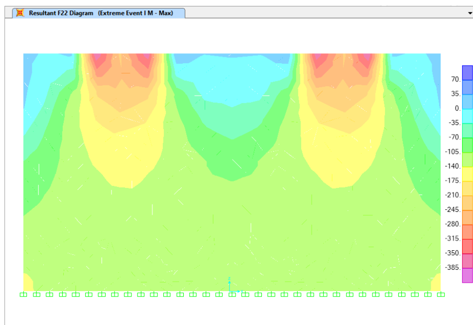
Figura 4.46: Fuerzas axiales máximas de Evento Extremo SAP2000. Fuente: Autores.
