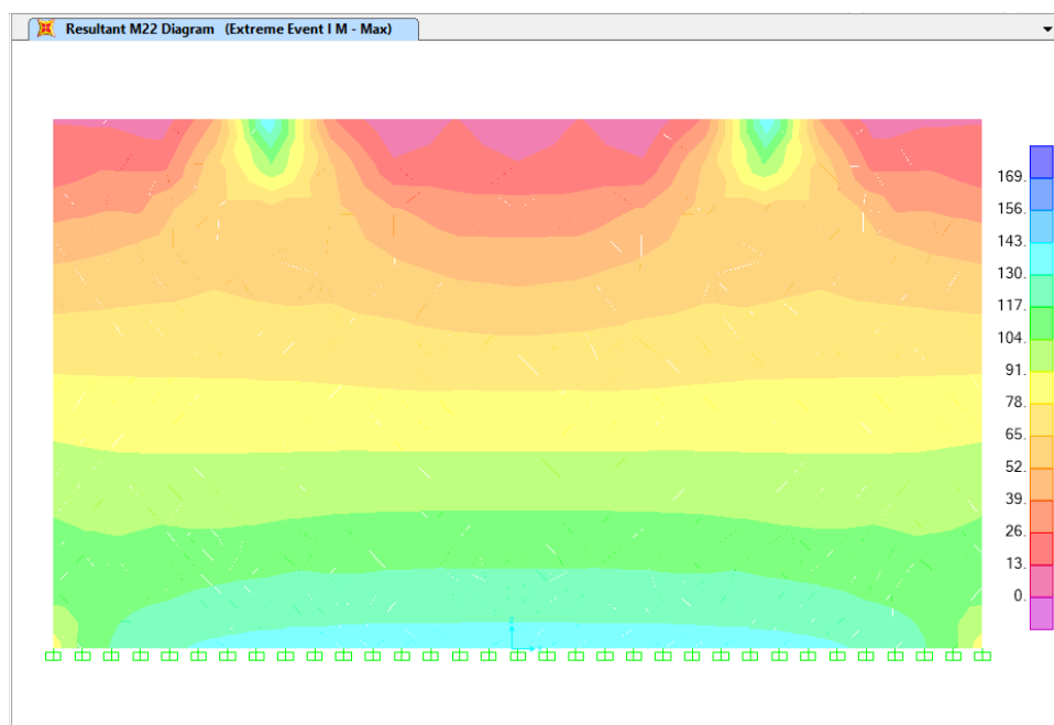
Figura 4.44: Momentos Máximos de Evento Extremo SAP2000. Fuente: Autores.
