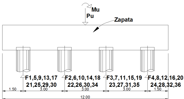
Figura 7.60: Distribución 2, lateral de los pilotes para la pila P3. Fuente: Autores.
