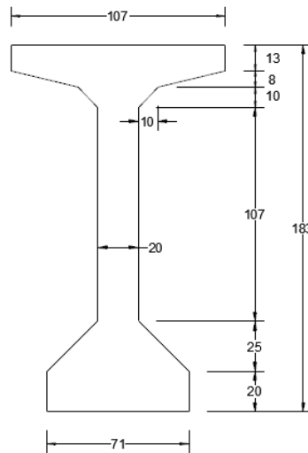
Figura 7.10: Viga AASHTO VI. Fuente: AASHTO.
