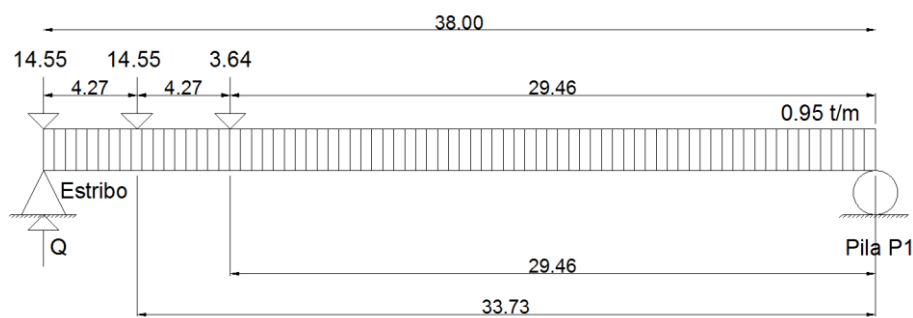
Figura 7.47: Ubicación longitudinal del camión de diseño.
