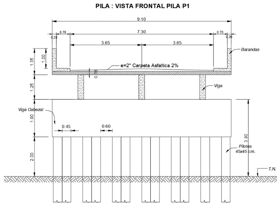
Figura 4.55: Vista frontal pila P1 del puente de Tarifa.
