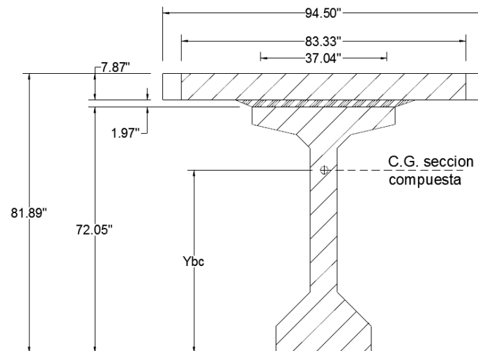
Figura 7.11: Viga AASHTO VI. Fuente: AASHTO.
