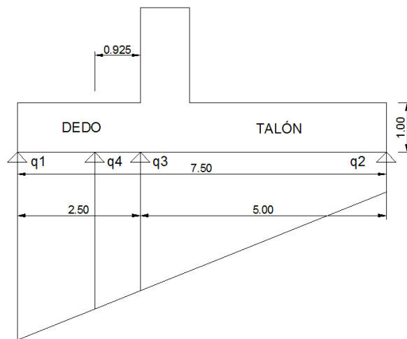
Figura 7.52: Distribucion de presiones para el dedo de la zapata. Fuente: Autores.
