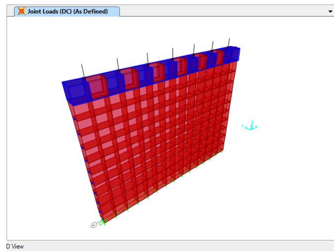
Figura 7.30: Ubicación de las cargas en pila 3 SAP2000.
