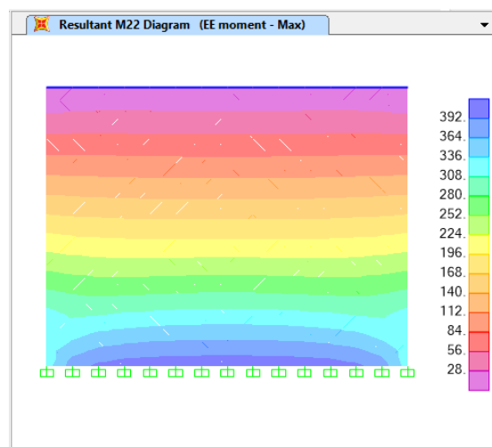
Figura 7.31: Momentos Máximos de Evento Extremo SAP2000.
