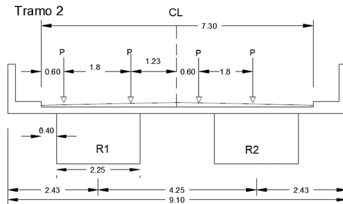
Figura 4.21: Sección transversal y ubicación de vehículos para momentos tramo 2. Fuente: Autores.
