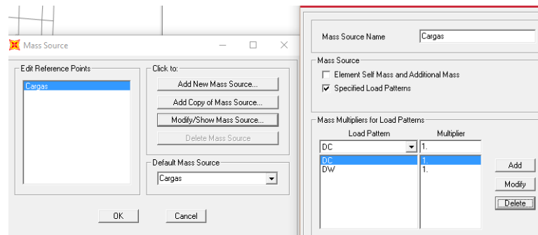
Figura 7.27: Definir fuente de masa por cargas SAP2000. Fuente: Autores.
