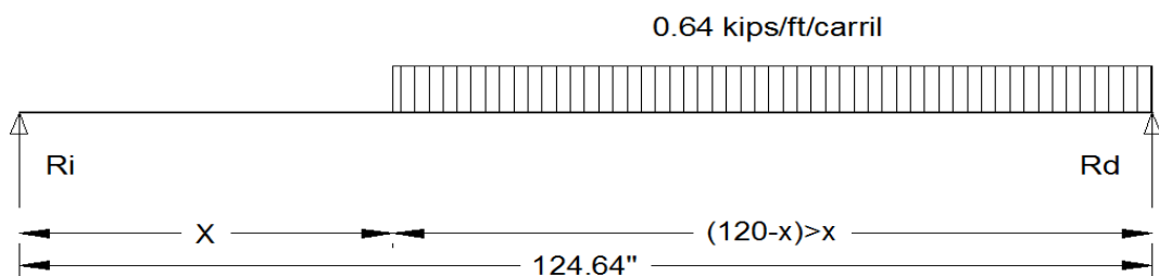
Figura 6.7: Modelo para obtención de cortantes máximos por carga de carril.
