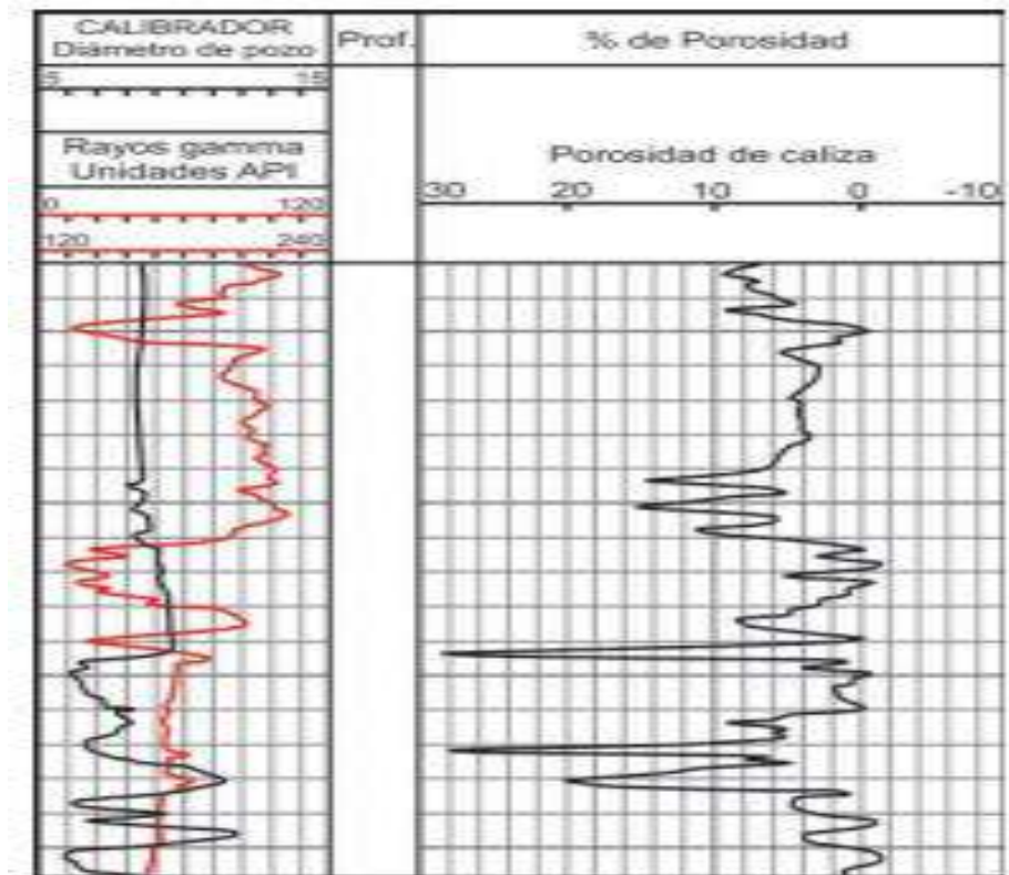
Figura 2.7 Registro neutrón tomado con la herramienta SNP.
