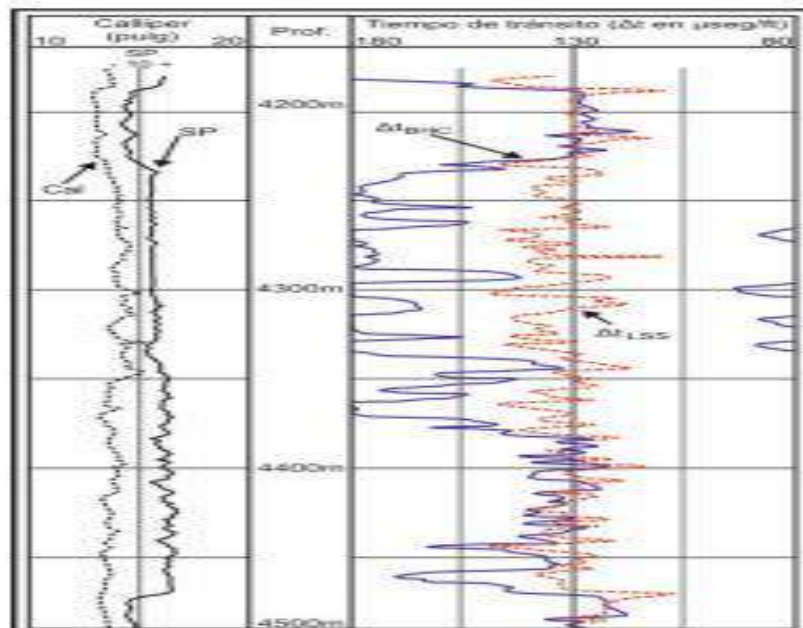
Figura 2.8 Ejemplo de un registro sónico de porosidad.
